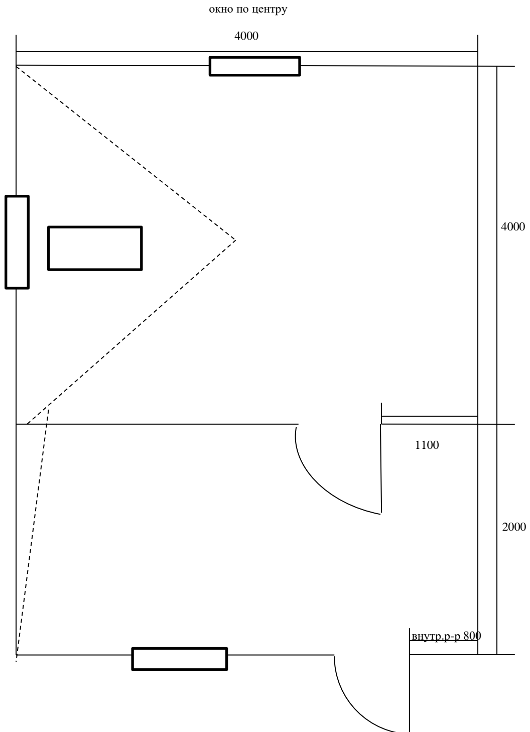
Арт 129 План-схема садового домика р-р 4000х4000 мм с верандой р-р 4000х2000 мм
