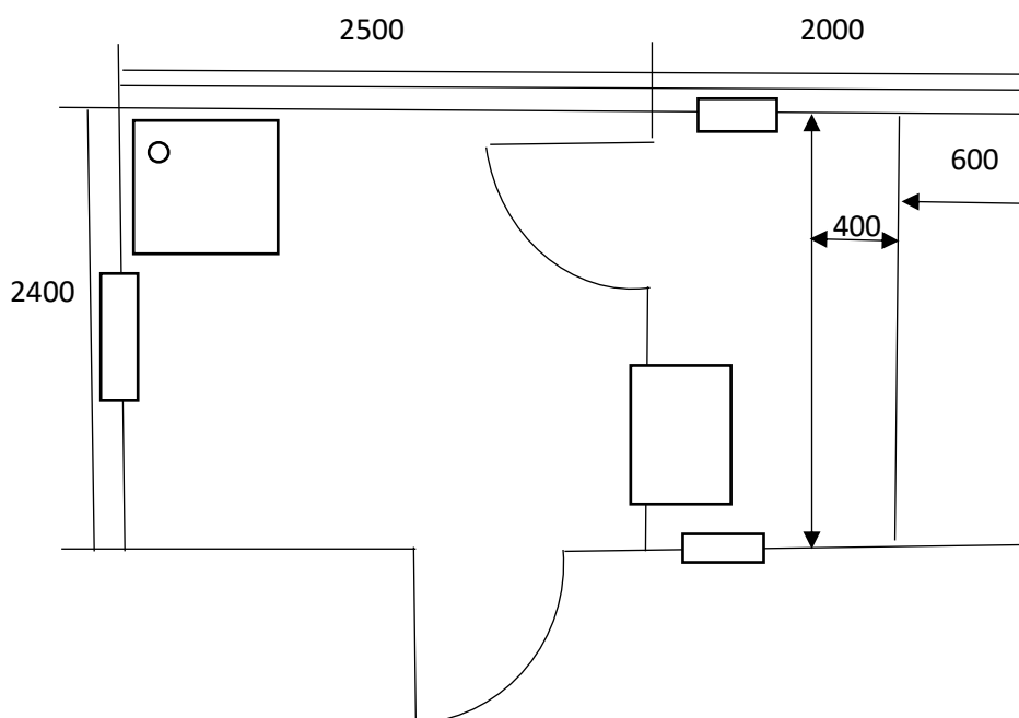
План-схема мобильной бани из блок-контейнера р-р 4500x2400 мм, арт. 143
