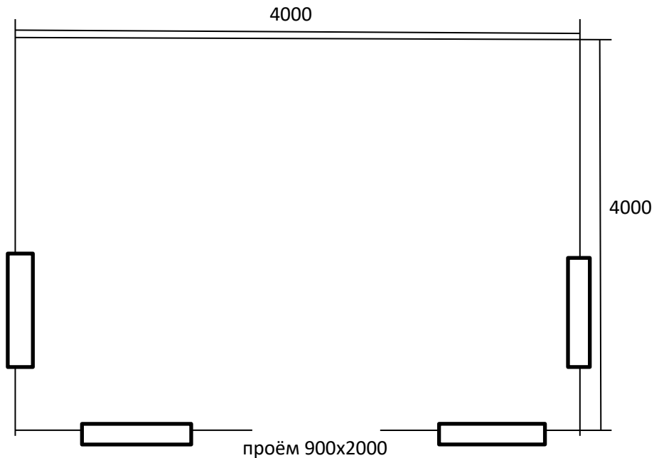
План-схема беседки р-р 4000х4000 мм
