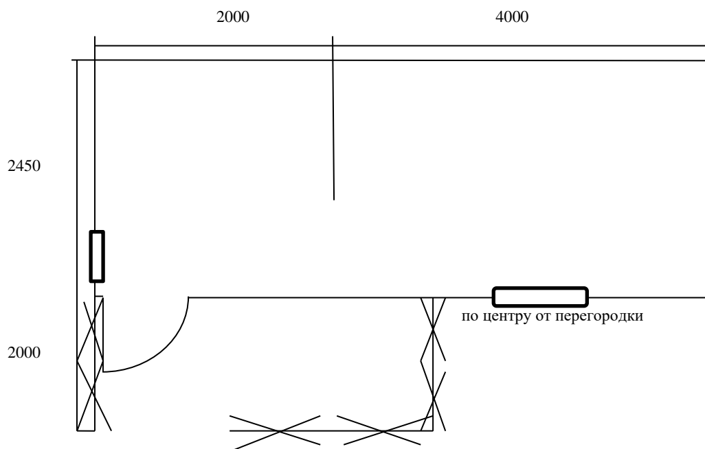
Спецификация на бытовку р-р 6000x2450 мм с террасой р-р 3000x2000 мм, арт. 157
