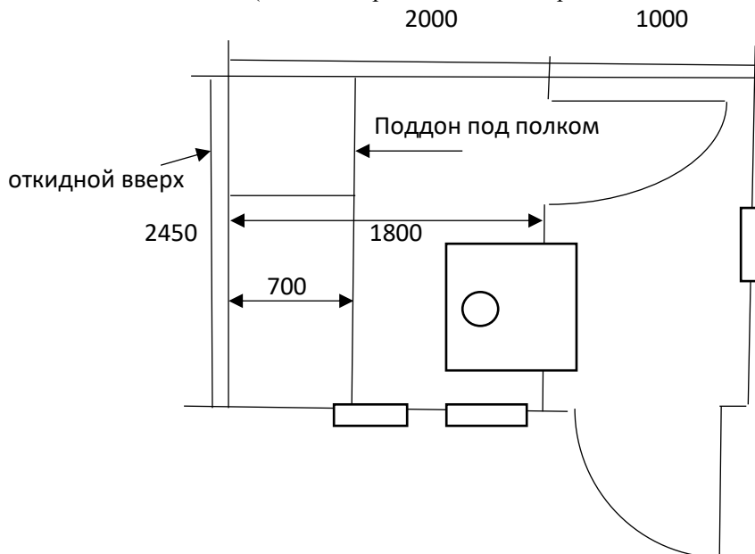
Арт. 276 План-схема мобильной деревянной бани-душ р-р 3000х2400 мм «Мал да удал» (изменение расположения дверок и окон на стоимость не влияет)
