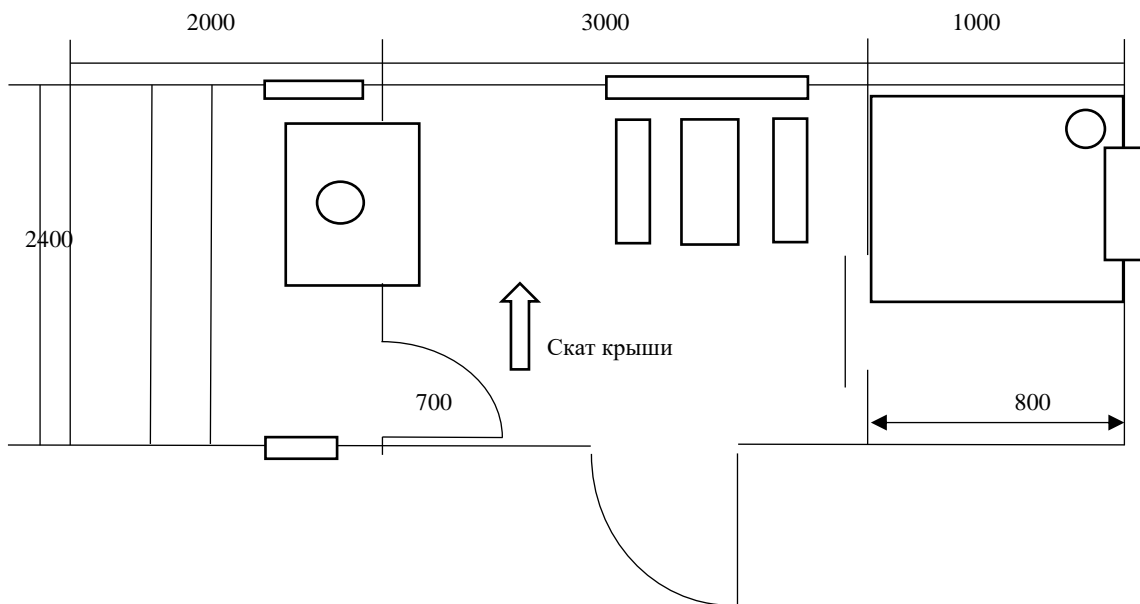
Спецификация на каркасную баню р-р 6000х2400 мм «Добрая банька», арт. 378
