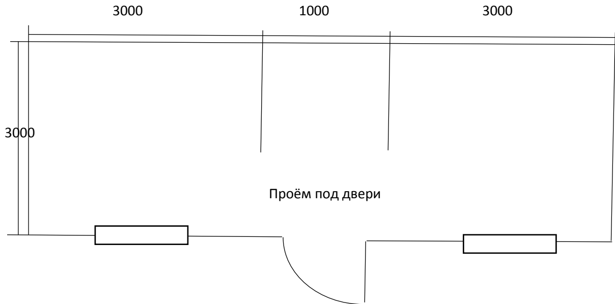
Спецификация на бытовку деревянную р-р 7000х3000 мм, арт.301
