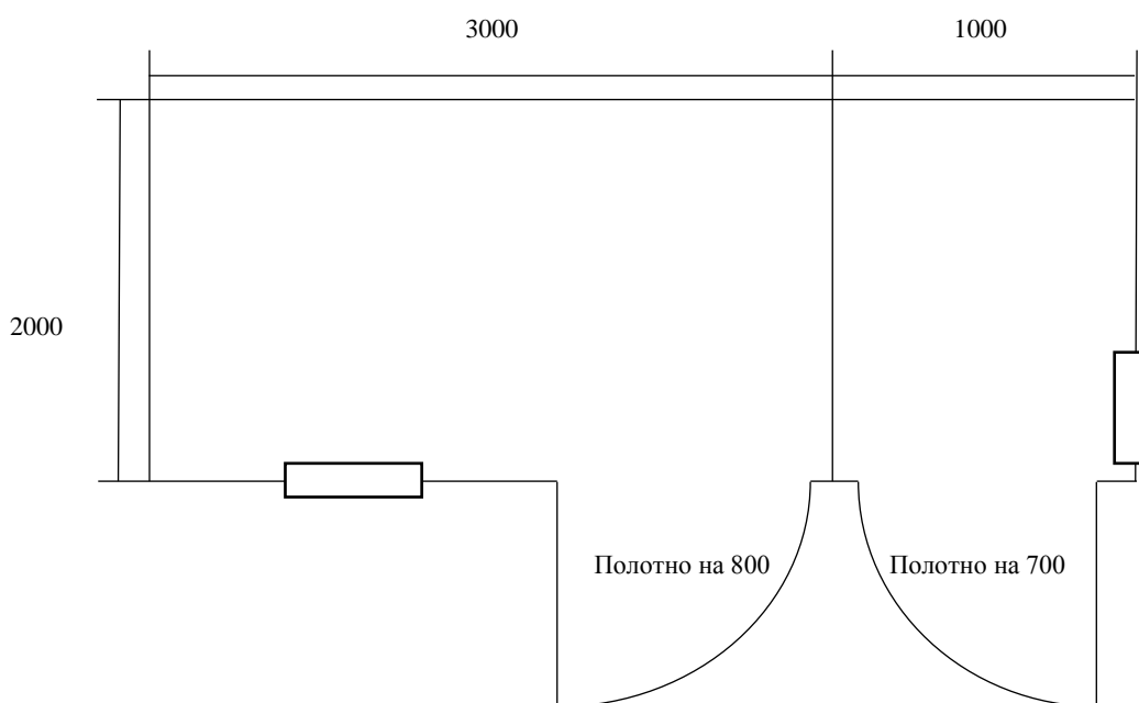
Спецификация на бытовку р-р 4000х2000 мм «Функционал», арт. 345
