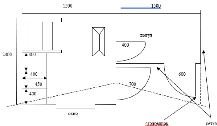
Курятник с выгулом р-р 3,0х2,4 "Грильяж" План-схема курятника с выгулом размера 3,0х2,4
